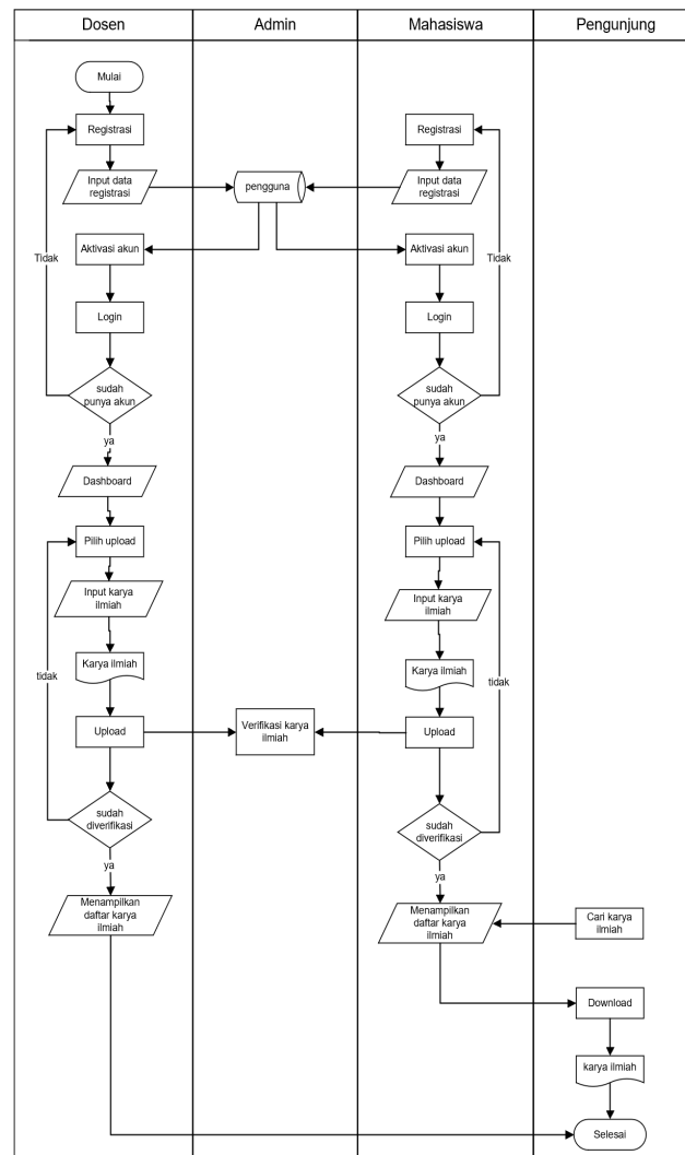
Gambar 2. Flowchart Sistem yang Diusulkan
